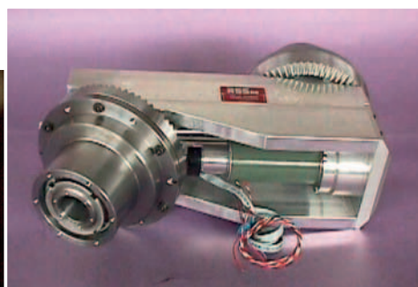
Bild 1. Das vordere Kronenrad sitzt unter einem Winkel von 68° auf dem Ritzel, das hintere unter 83° – eine Anordnung, die mit Kegeln nicht möglich ist
